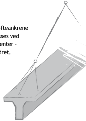
Figur: Løft enkelt ribbet tagplade
