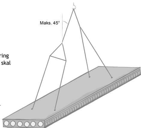
Figur: Løft huldæk
