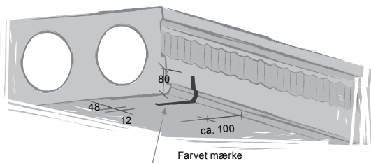
Figur: Vederlag huldæk
