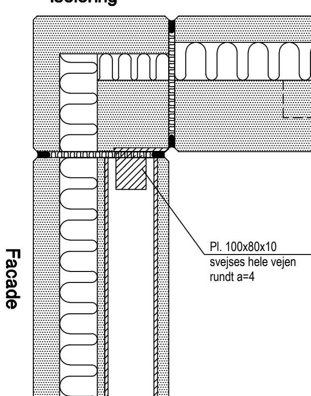
Snit A-A
