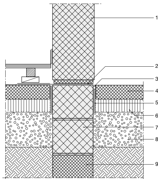
Eksempel: Enkeltvæg ved fundament Luftlydisolation: R'_w \geq 55 dB
