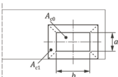
Figur 6.2 Symmetrisk 4-sidig lastfordeling for last placeret med afstand til kanter baseret på afstanden til nærmeste kantafstand
