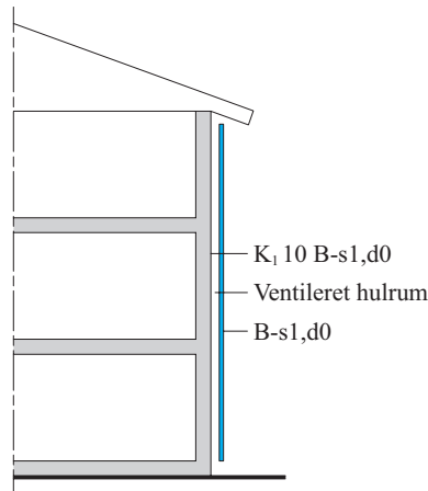
Figur 5.3. Regnskærm.
