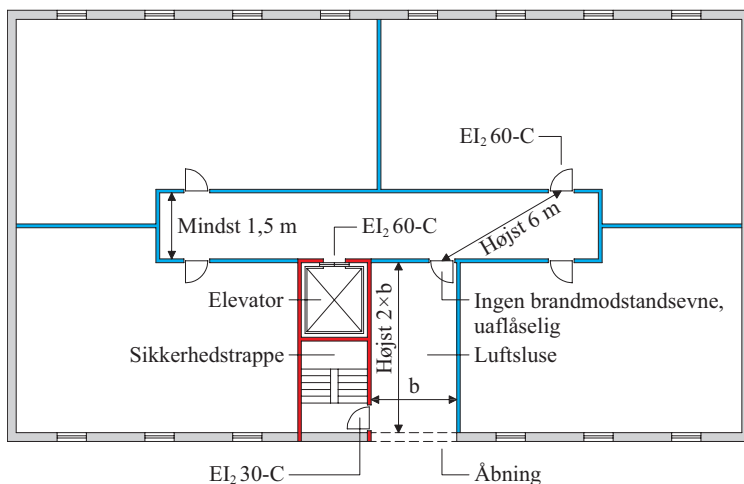
Figur 2.11. Luftsluse og sikkerhedstrappe.
