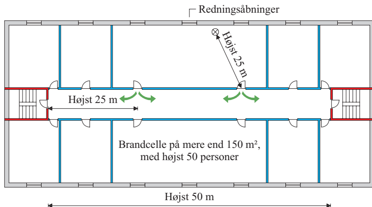
Figur 2.1. Døre til flugtveje fra brandcelle over 150 m² og med højst 50 personer.
