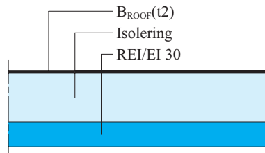
Figur 3.3. Tagkonstruktion.
