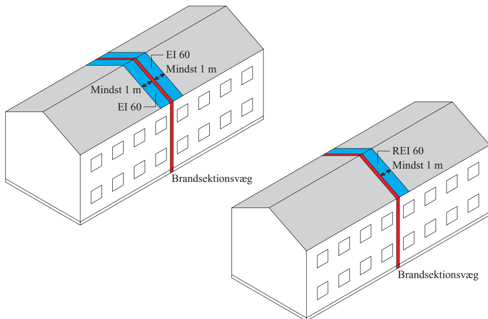
Figur 5.7. Brandkamserstatning.
