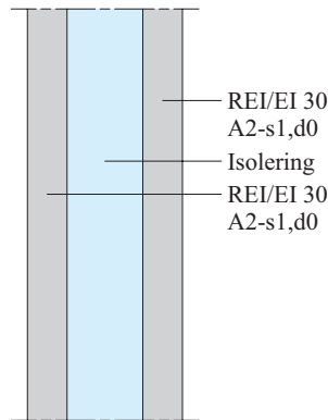
Figur 3.2. Lodret bygningsdel.
