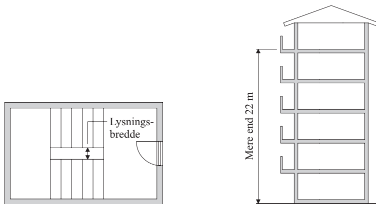
Figur 6.4. Lysningsbredde.
